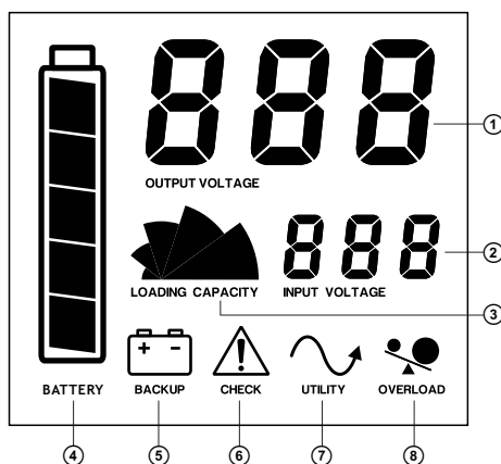
Рис. 1. LCD-дисплей ИБП
