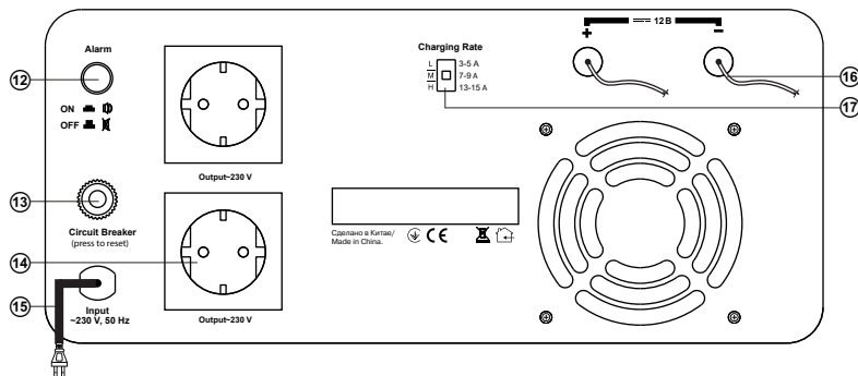
Рис. 3. Задняя панель RT-1000
